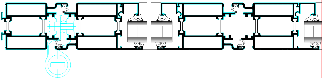
Porte à l'anglaise à deux vantaux
