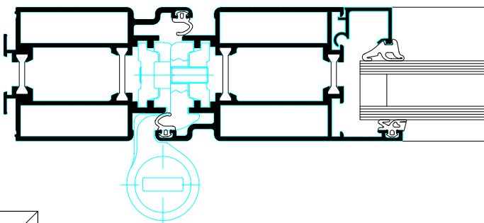
Porte à l'anglaise à deux vantaux
